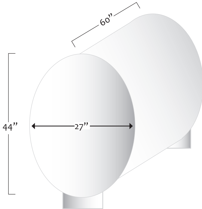
275 gallon capacity 718G--27500 AG
